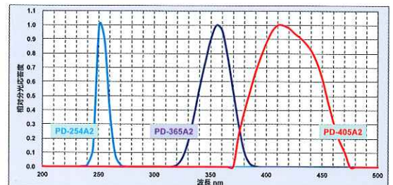
各受光部の相対分光応答度
